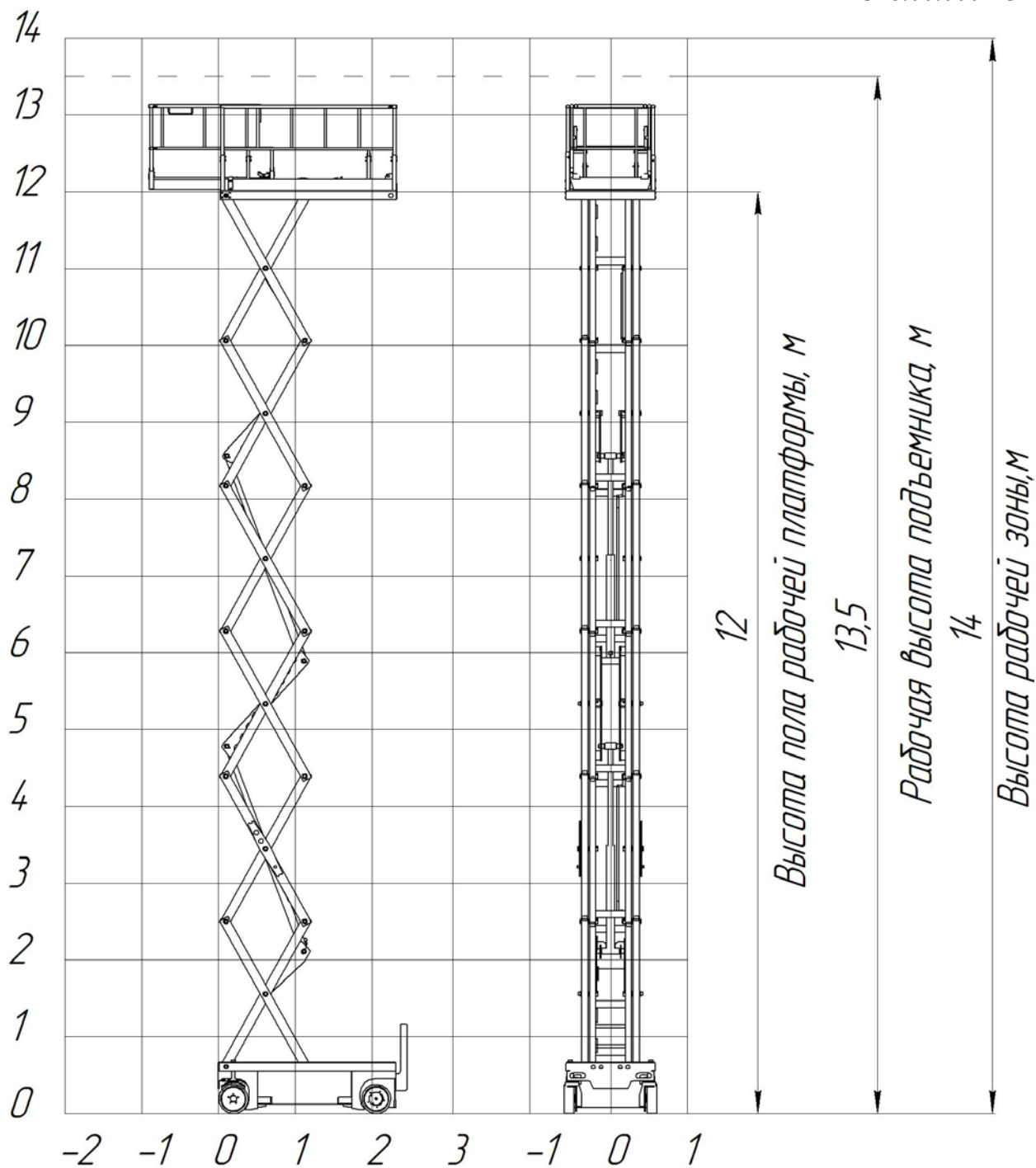
Рисунок А5 – Высотные характеристики подъемника ЭЖО14
