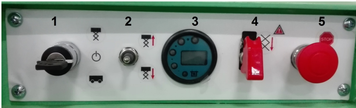
Рис 7 - Пульт управления на шасси (нижний пульт)
